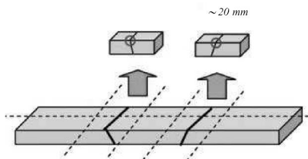
Fig. 2.6.8.3.1.1.1 Sectioning plan
